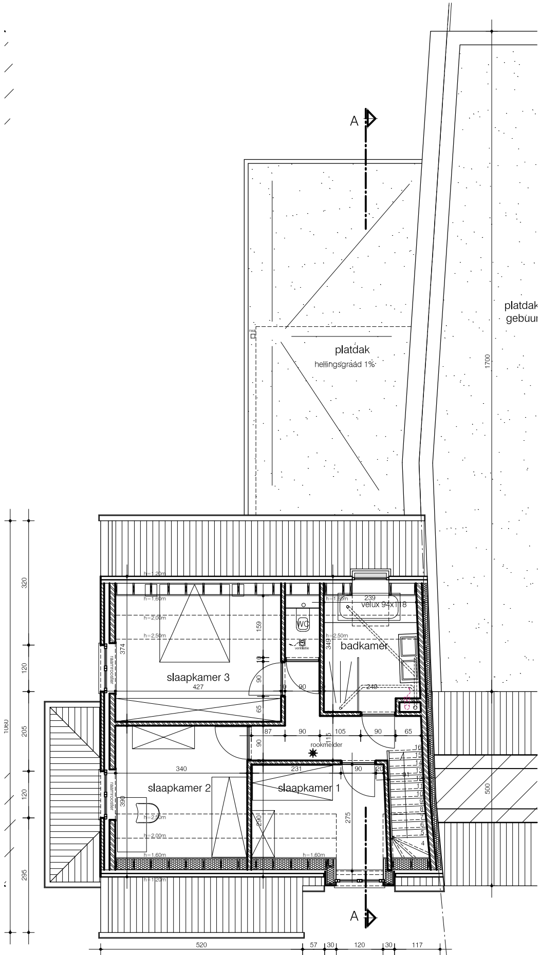
GRONDPLAN EERSTE VERDIEPING
