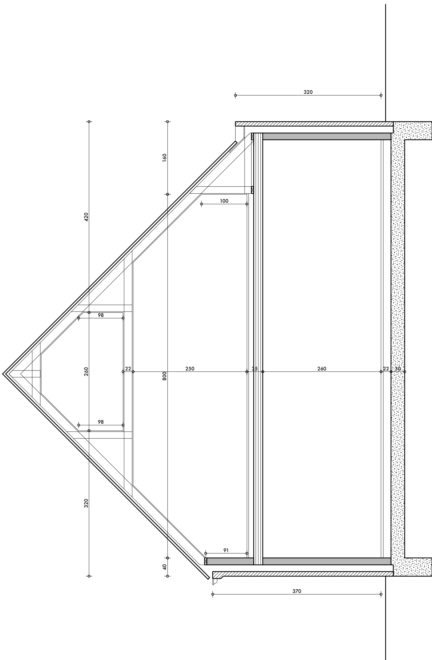
PRINCIPESNEDE SCHAAL 1 - 50
